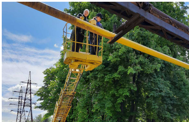
На високих ділянках трубопроводу застосовуємо автокран
